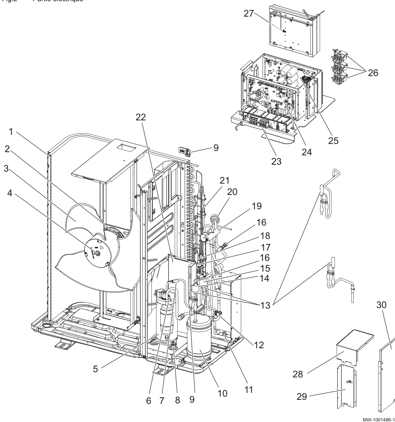
Fig.2 Partie électrique
