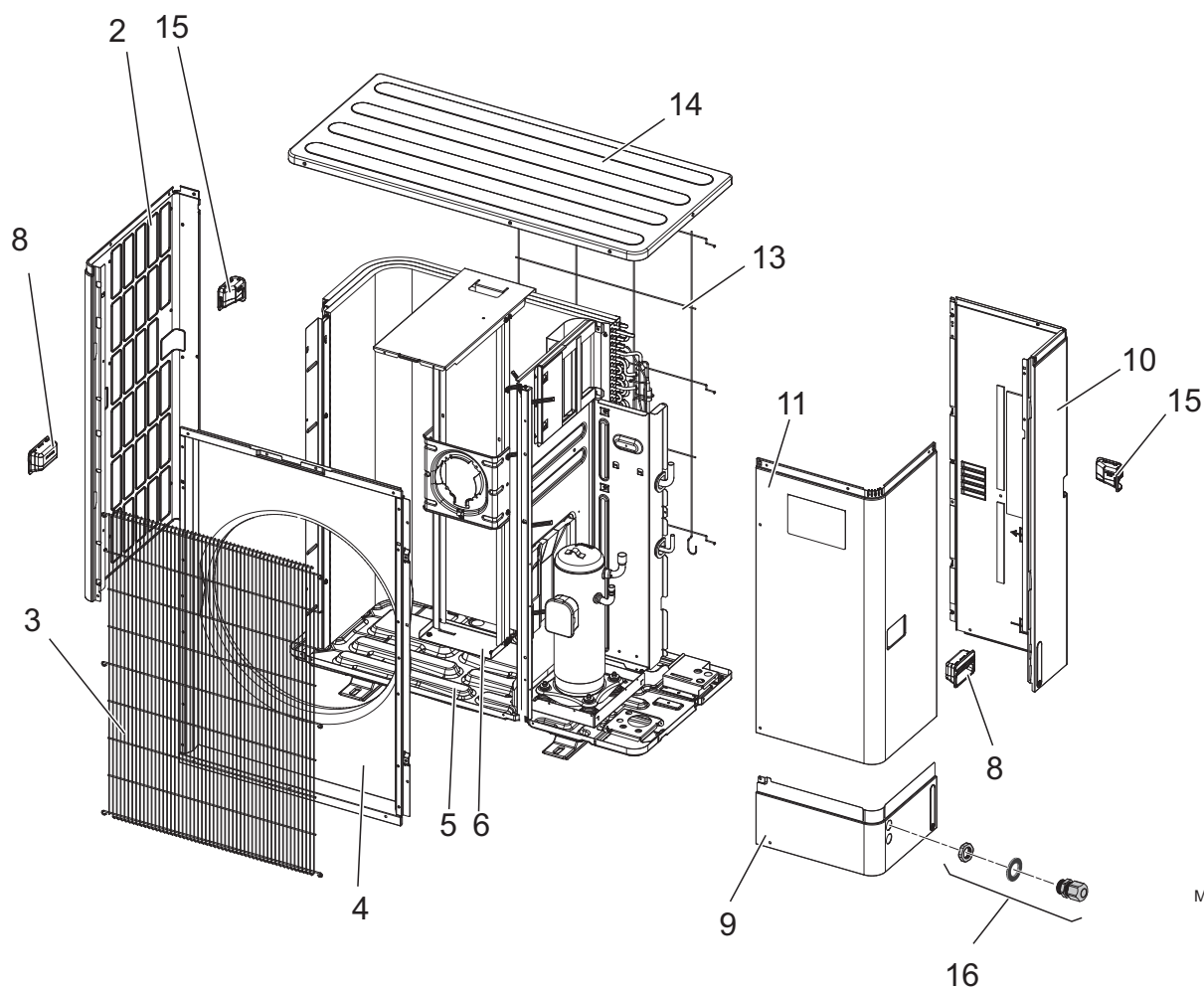
Fig.7 Châssis
