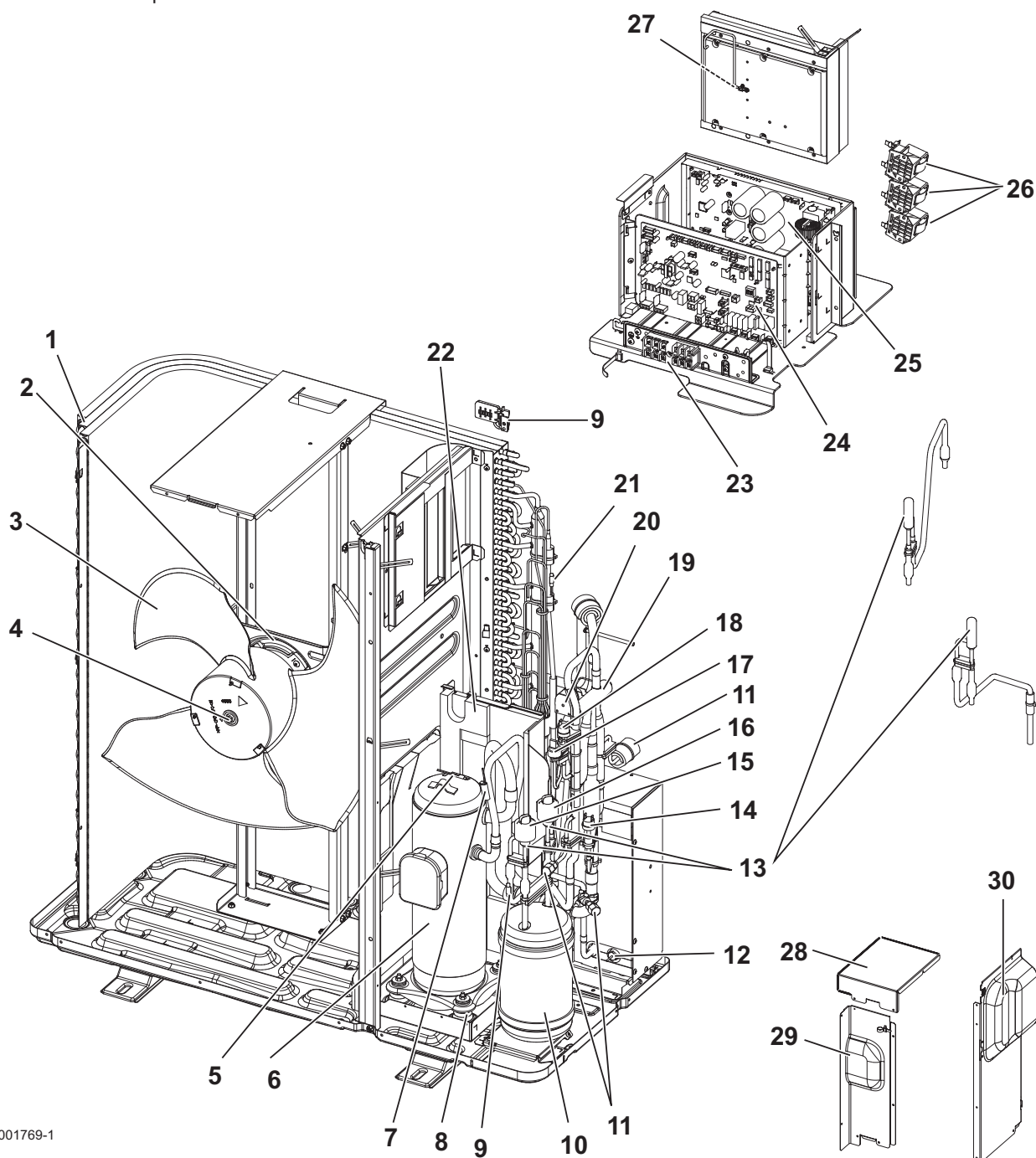
Fig.6 Partie électrique
